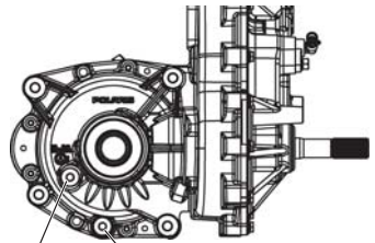
Einfüllschraube Ablassschraube
